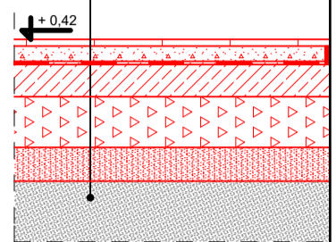
Przekrój B-B skala 1:20
