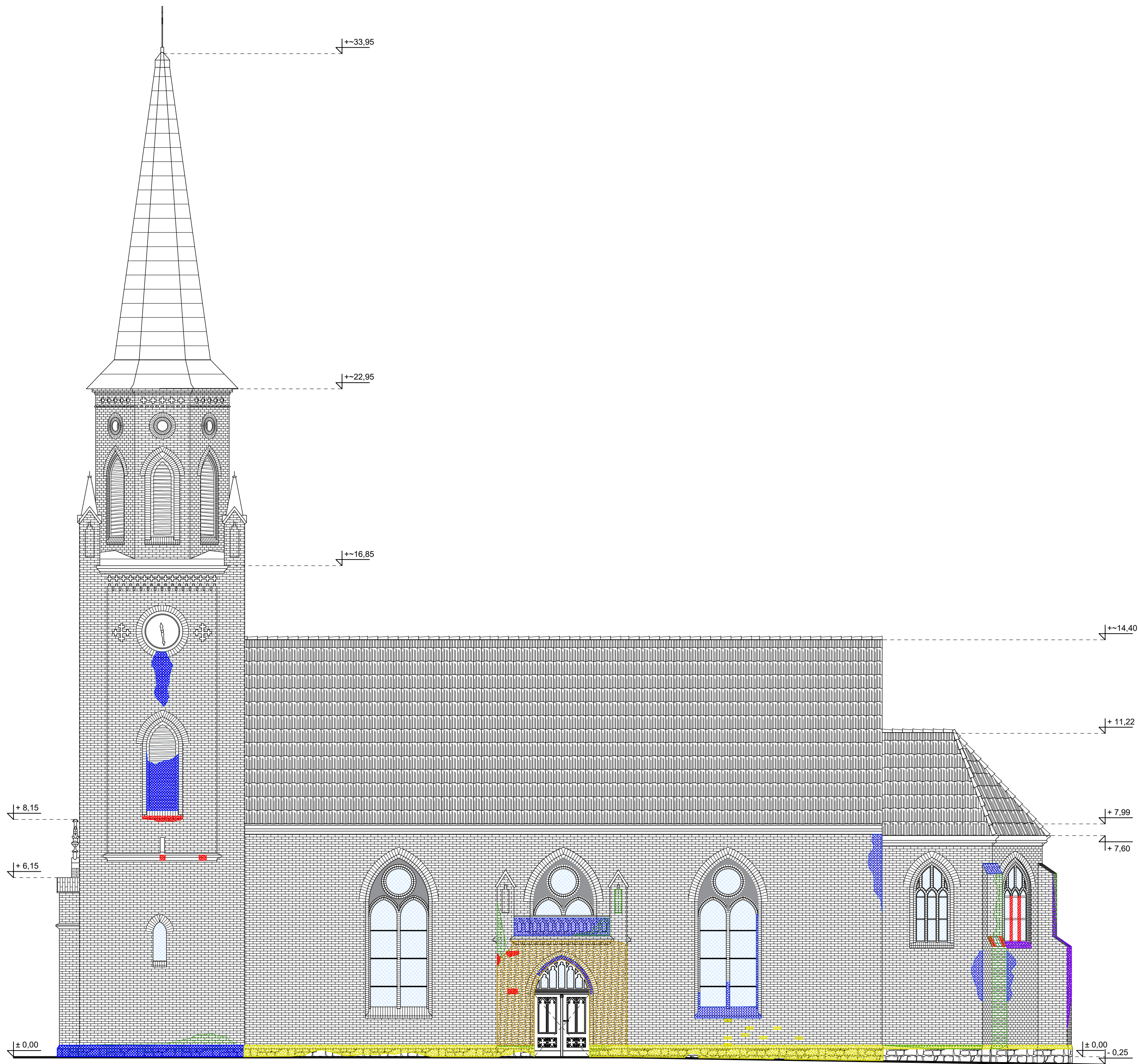
ELEWACJA POŁUDNIOWA
