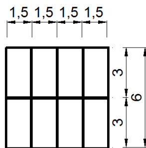
Rys.2. Schemat układania płyt na drogach o dwóch pasach ruchu
